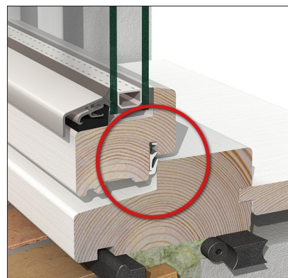
Q-Lon tætningsliste
